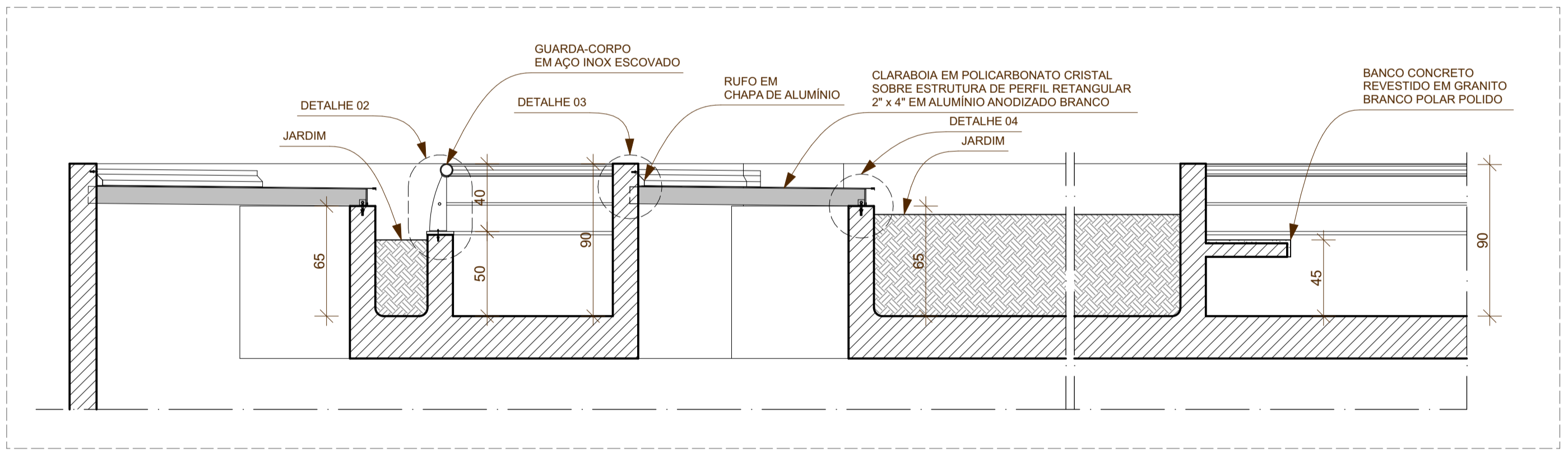
16 CORTE AA' 1:25
