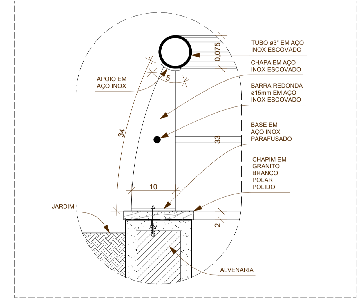
16 DETALHE 02 1:5
