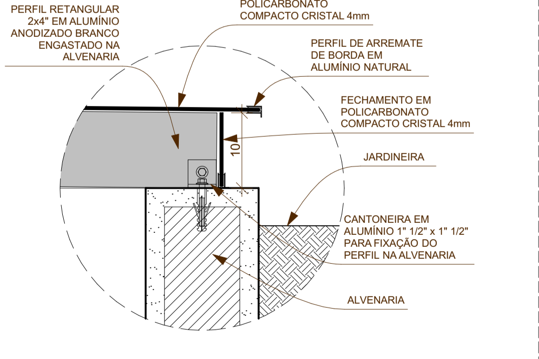
16 DETALHE 04 1:5
