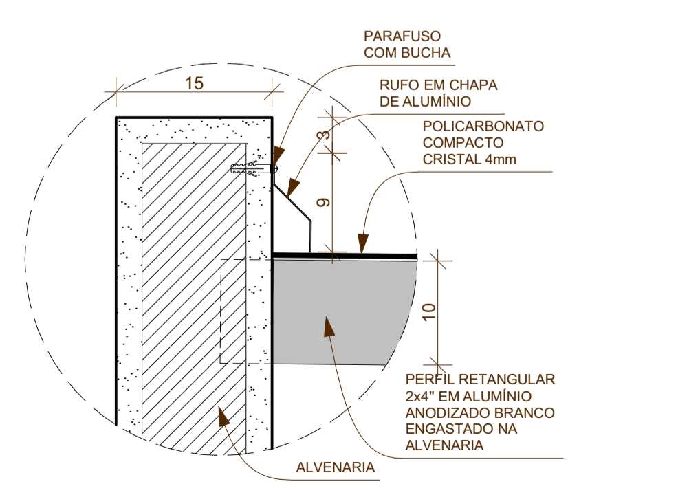
16 DETALHE 03 1:5
