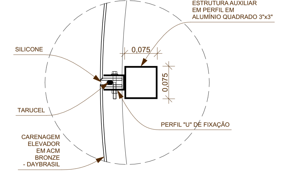
16 DETALHE 06 1:5
