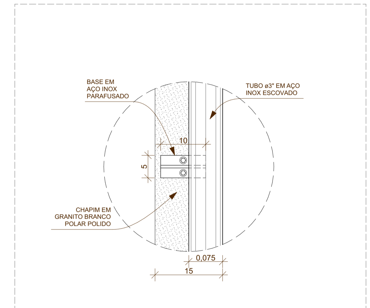
16 DETALHE 01 1:5
