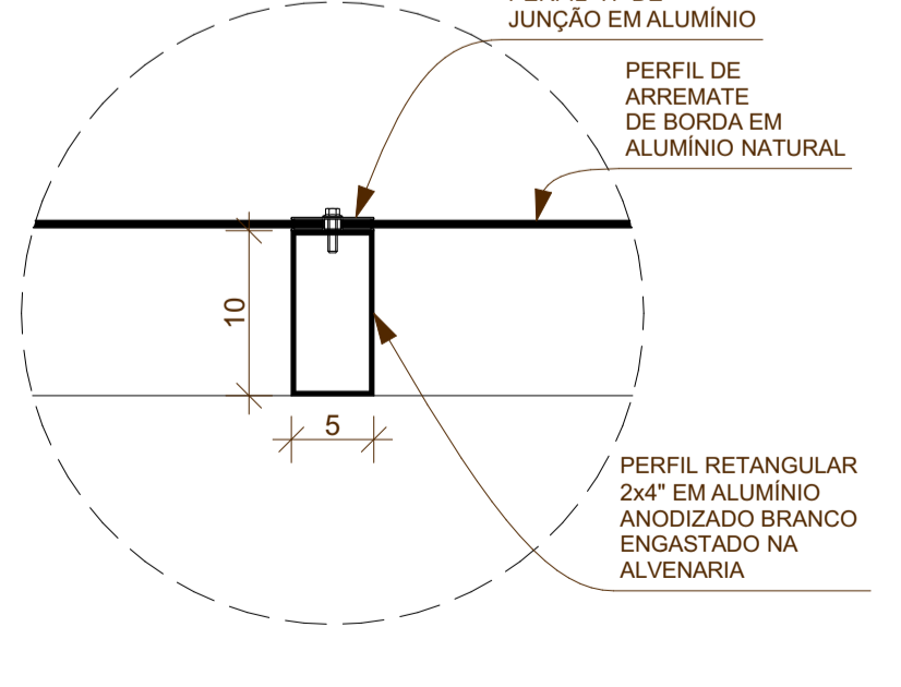
16 DETALHE 05 1:5
