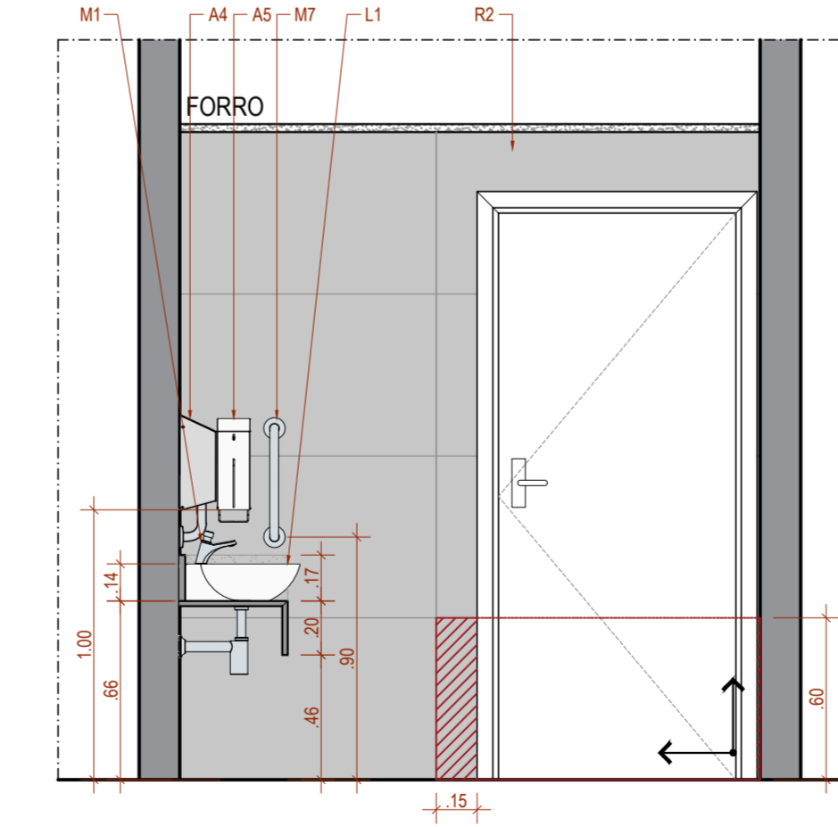
DETALHE GÊNÉRICO WC PNE COM BANCADA VISTA C
