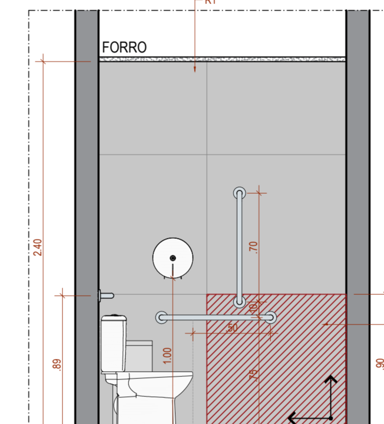
DETALHE GÊNÉRICO WC PNE SEM BANCADA VISTA C
