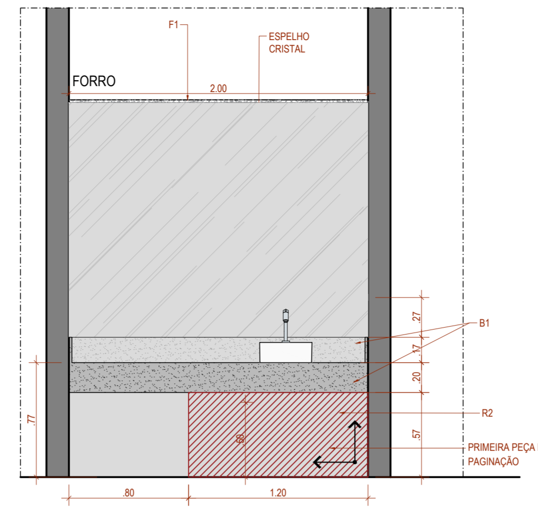
DETALHE GÊNÉRICO WC DO DEPUTADO COM BANCADA VISTA B
