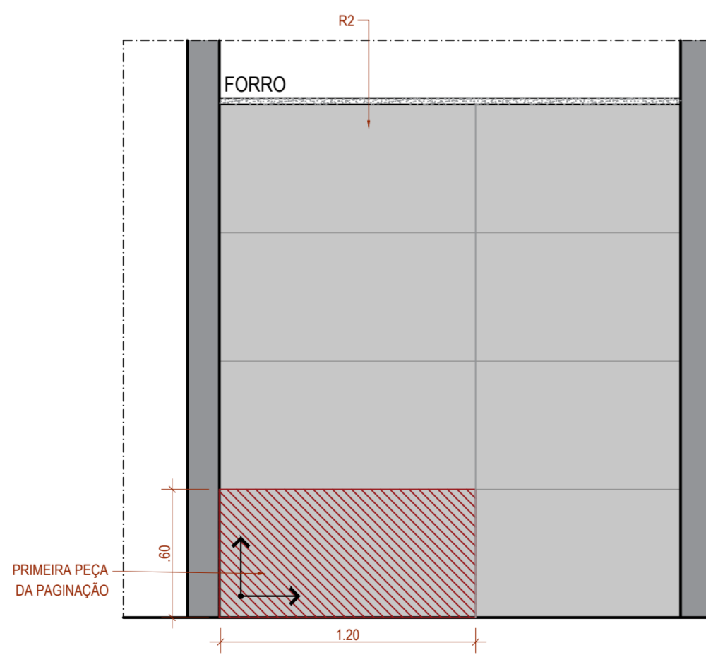
DETALHE GÊNÉRICO WC PNE COM BANCADA VISTA A
