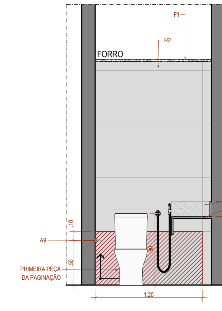
DETALHE GÊNÉRICO WC DO DEPUTADO COM BANCADA VISTA D
