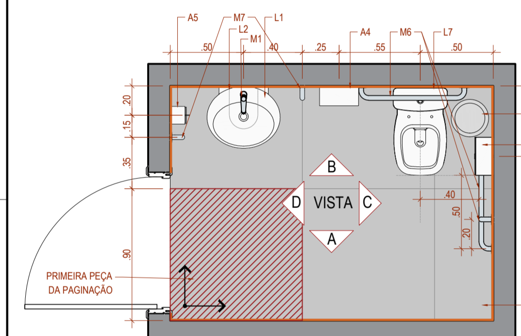
DETALHE GÊNÉRICO WC PNE SEM BANCADA PLANTA BAIXA
