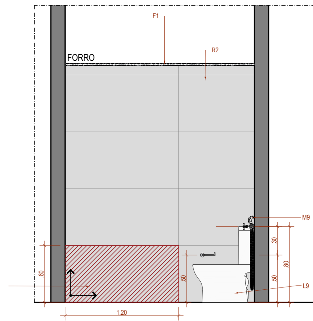
DETALHE GÊNÉRICO WC DO DEPUTADO COM BANCADA VISTA A
