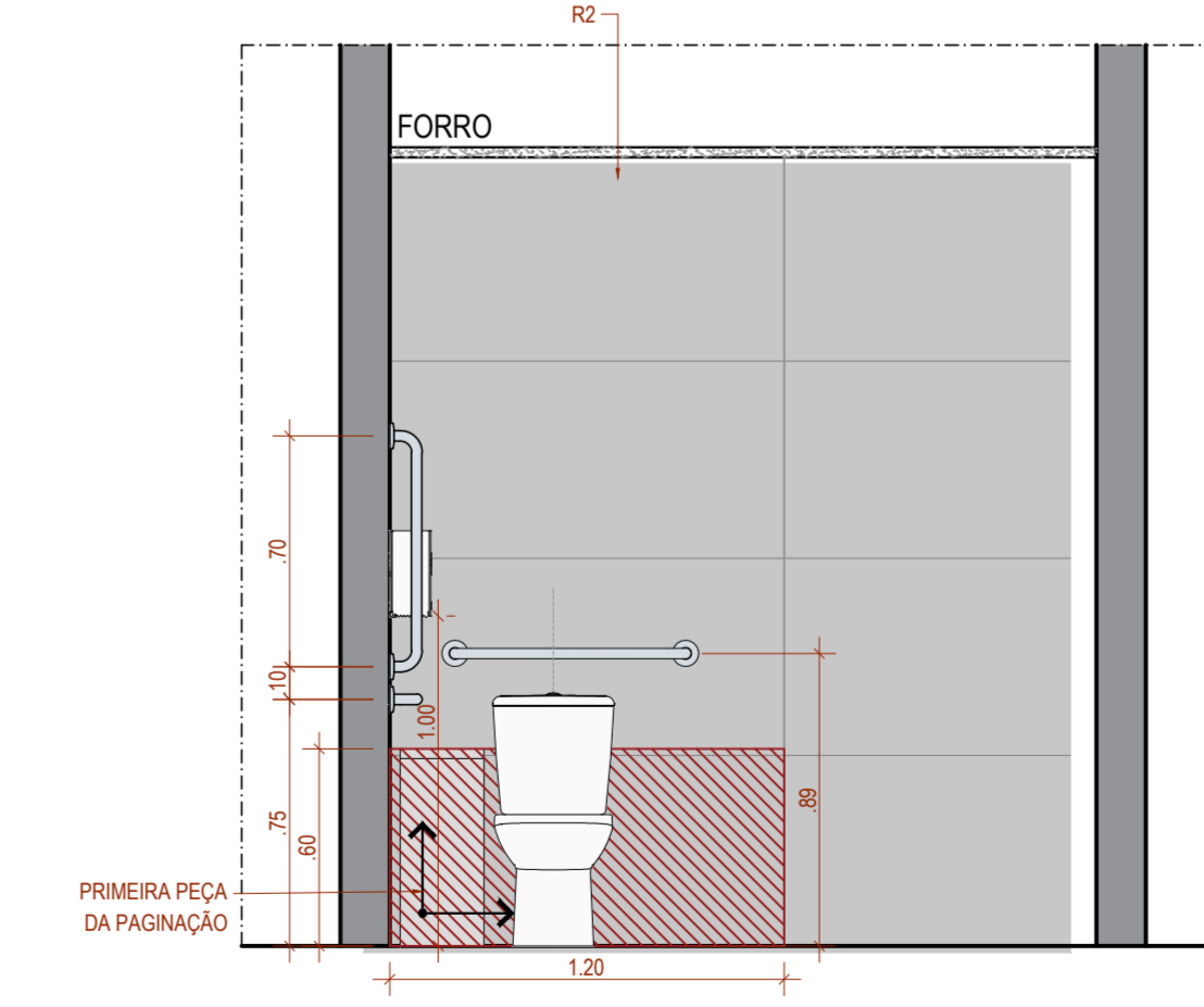
DETALHE GÊNÉRICO WC PNE COM BANCADA VISTA D
