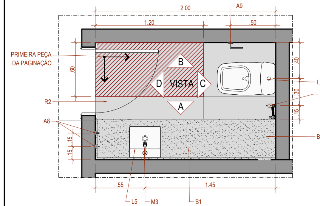
DETALHE GÊNÉRICO WC DO DEPUTADO COM BANCADA PLANTA BAIXA
