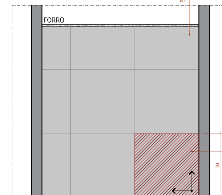
DETALHE GÊNÉRICO WC PNE SEM BANCADA VISTA A
