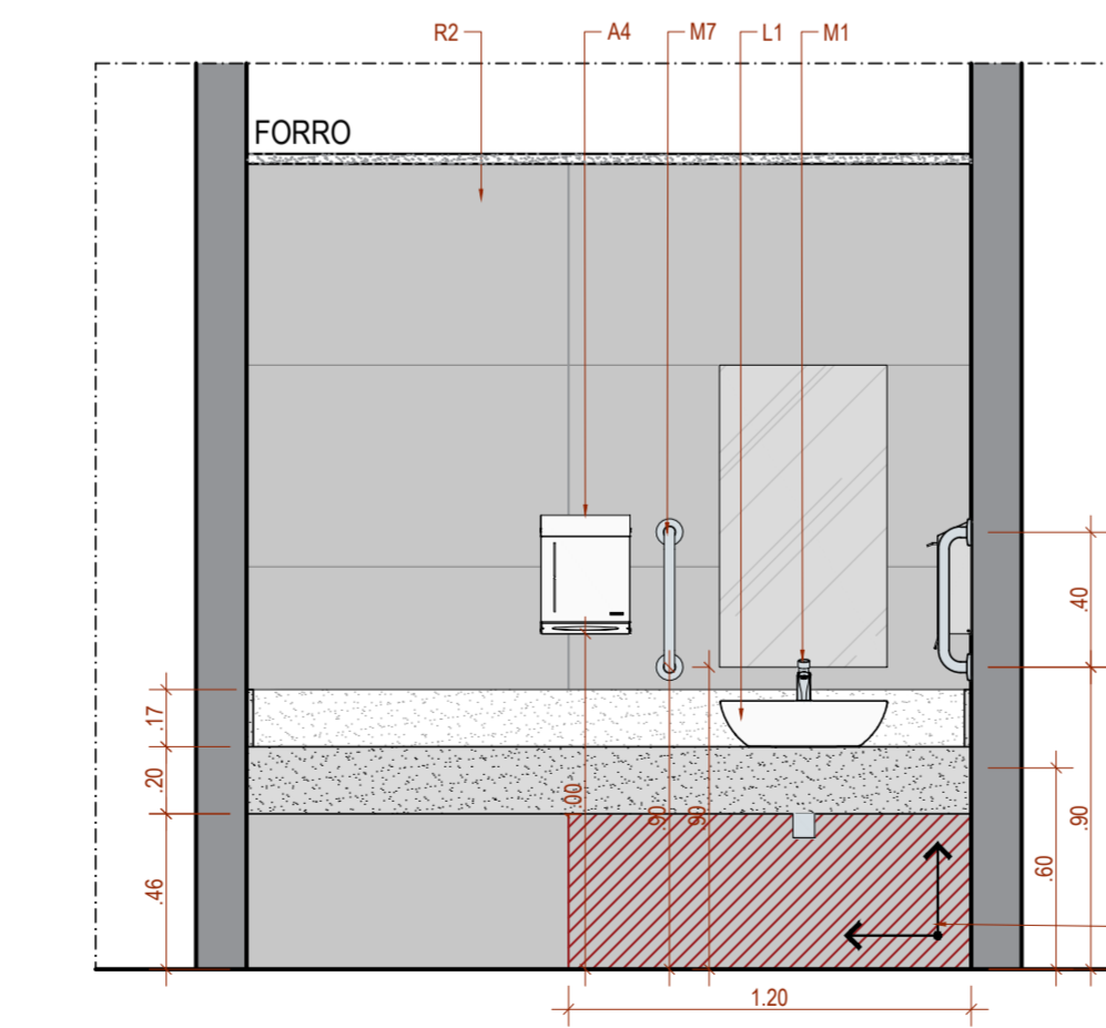
DETALHE GÊNÉRICO WC PNE COM BANCADA VISTA B
