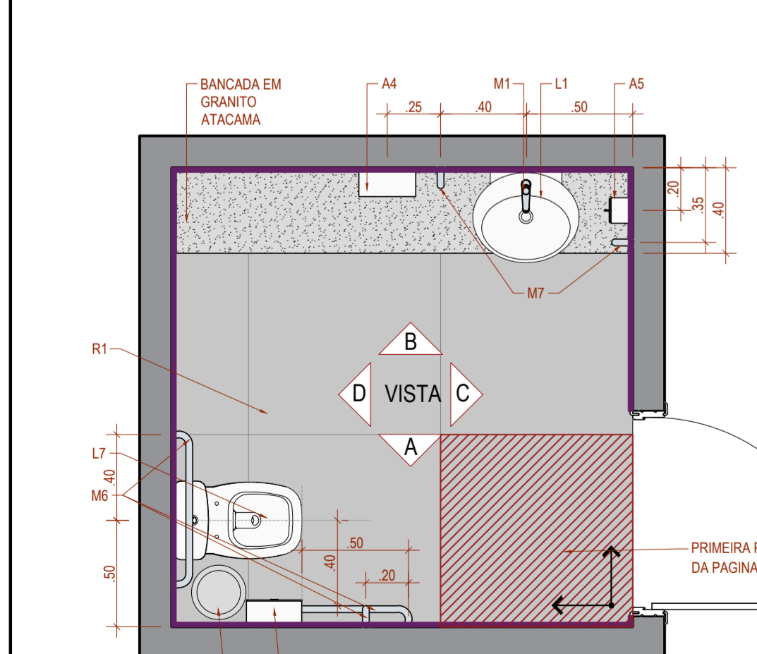
DETALHE GÊNÉRICO WC PNE COM BANCADA PLANTA BAIXA
