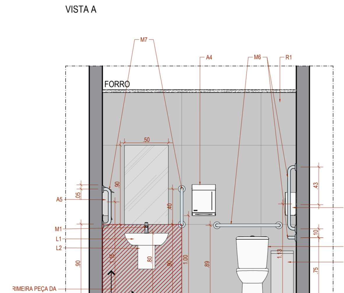
DETALHE GÊNÉRICO WC PNE SEM BANCADA VISTA B
