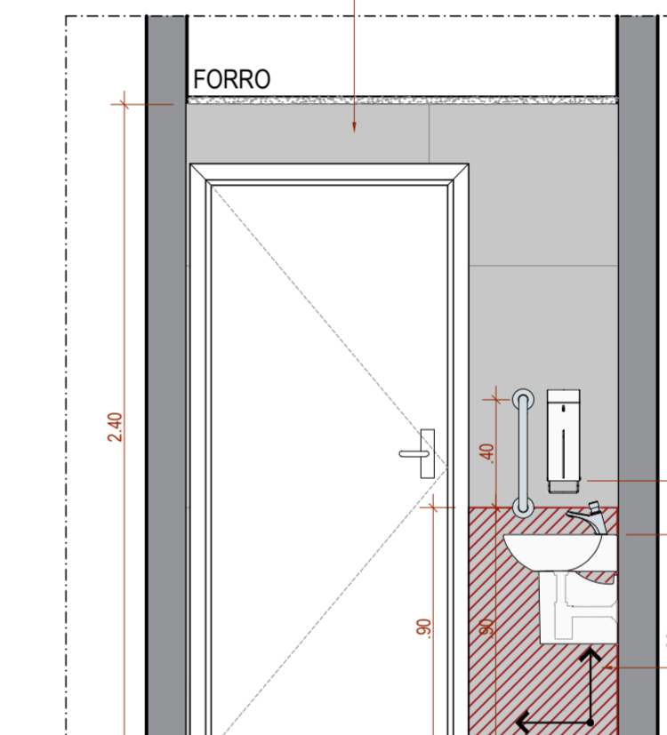
DETALHE GÊNÉRICO WC PNE SEM BANCADA VISTA D
